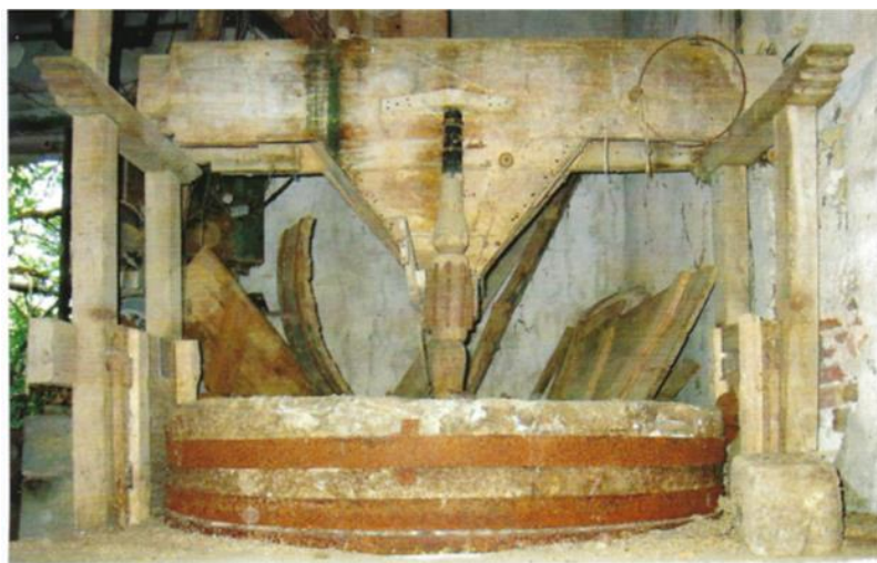
Moulin de la Dame : les meules et la trémie, système d'alimentation en grain. Et le Cavalet.
