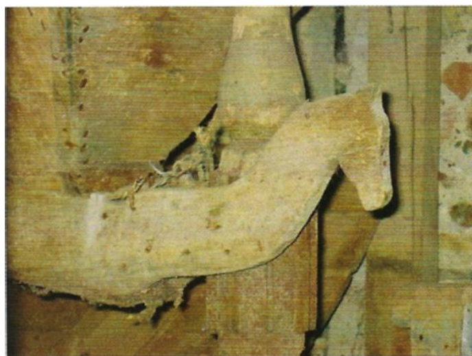
Moulin de la Dame : les meules et la trémie, système d'alimentation en grain. Et le Cavalet.
